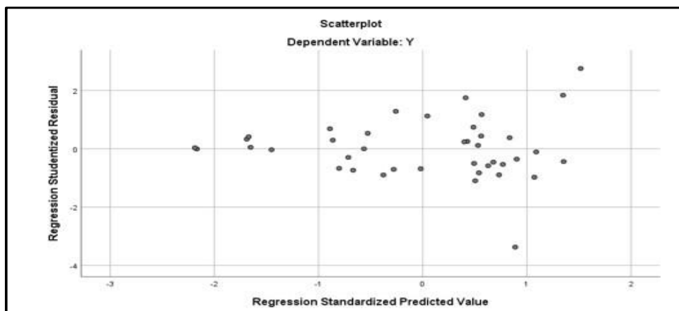
Gambar 2 Grafik Scatterplot
